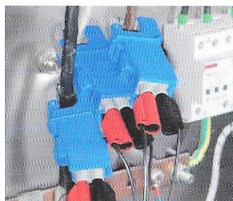
CT단자용 전류센서: 25mA~5A AC (A 1122+A1561)
